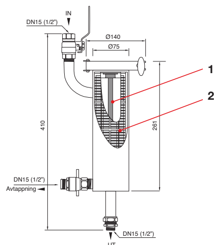
1. Magnetstav
